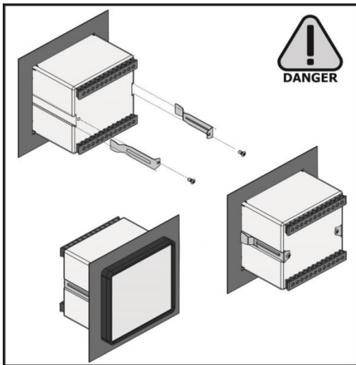
نصب Figure 1
